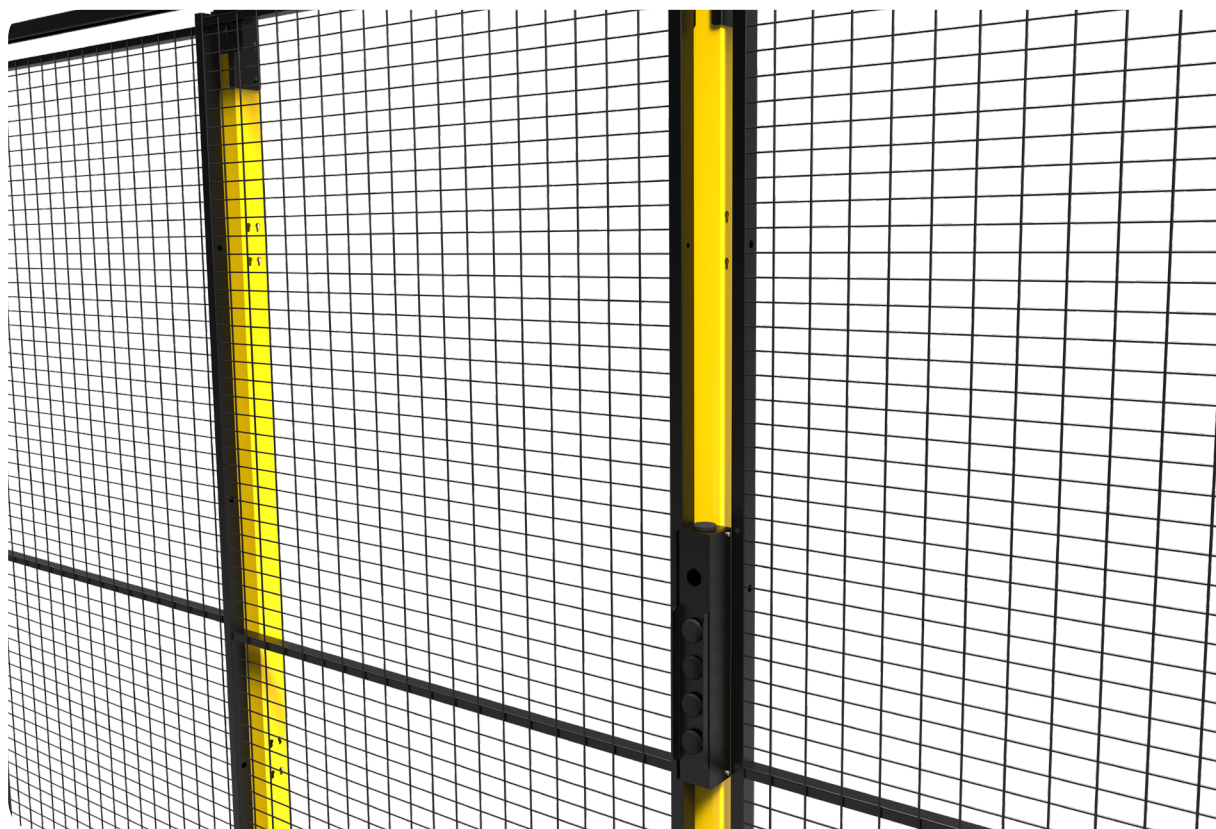
Tryckknappslåda monterad på stolpe vid skjutport.
